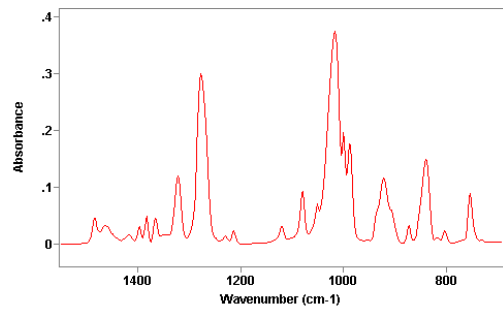
FTIR Spectrum
