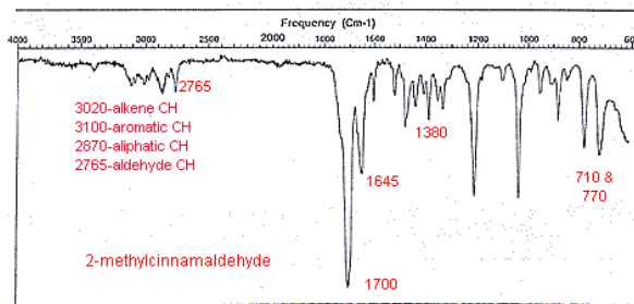
FTIR Spectrum
